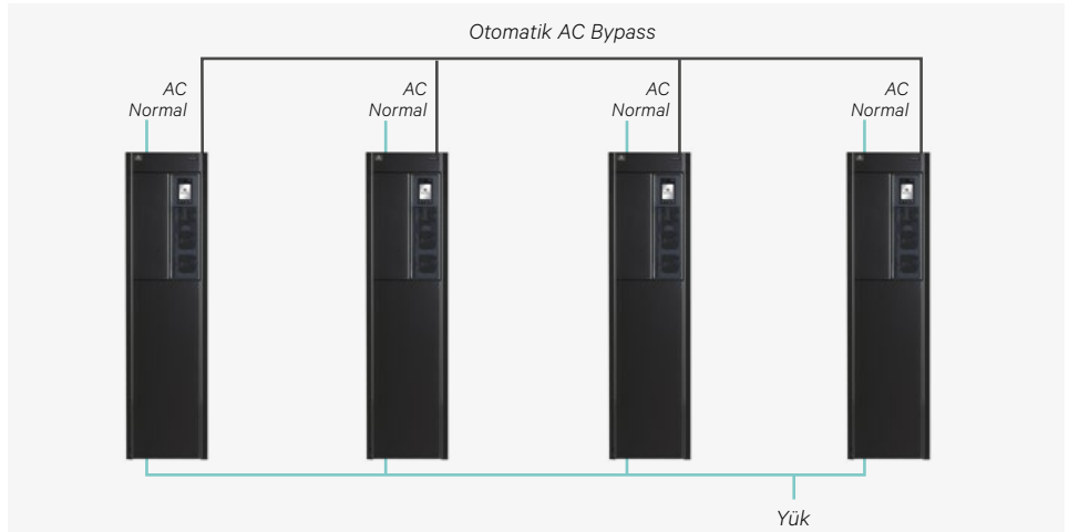
Liebert EXS - Paralel konfigürasyon
